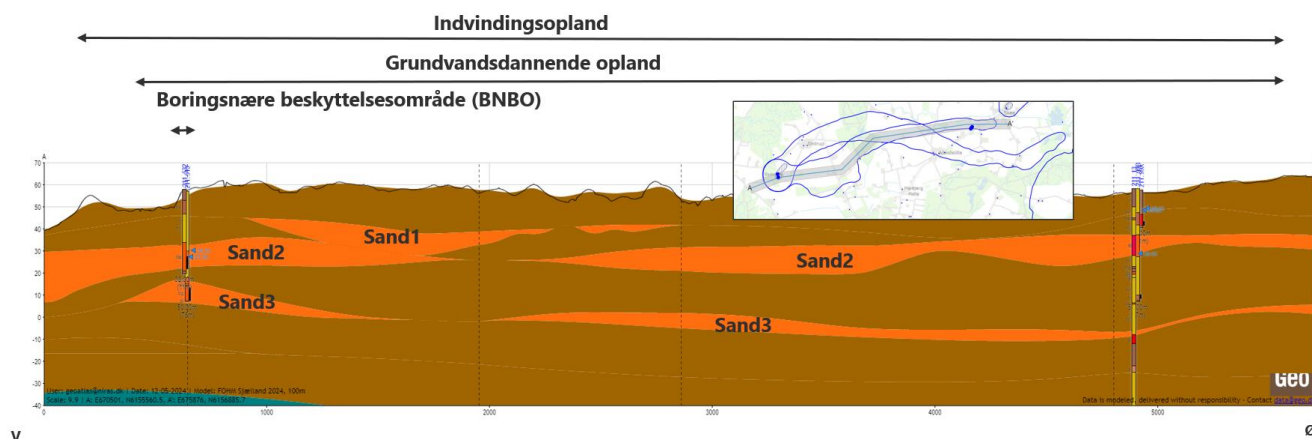
Figur 55 Geologisk profil gennem kildepladsen til DGU nr. 211.532. Brune og blå farver repræsenterer vandstandsene og oftest lerede aflejringer, orange farver repræsenterer vandførende aflejringer, typisk sand og grus.
