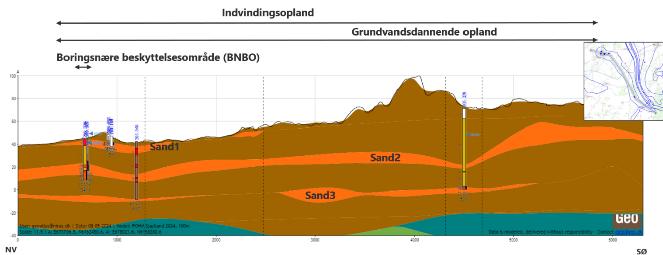
Figur 12 Geologisk profil gennem den vestlige kildeplads ved Kirke Eskilstrup by. Brune og blå farver repræsenterer vandstandsede og oftest lerede aflejringer, orange farver repræsenterer vandførende aflejringer, typisk sand og grus.
