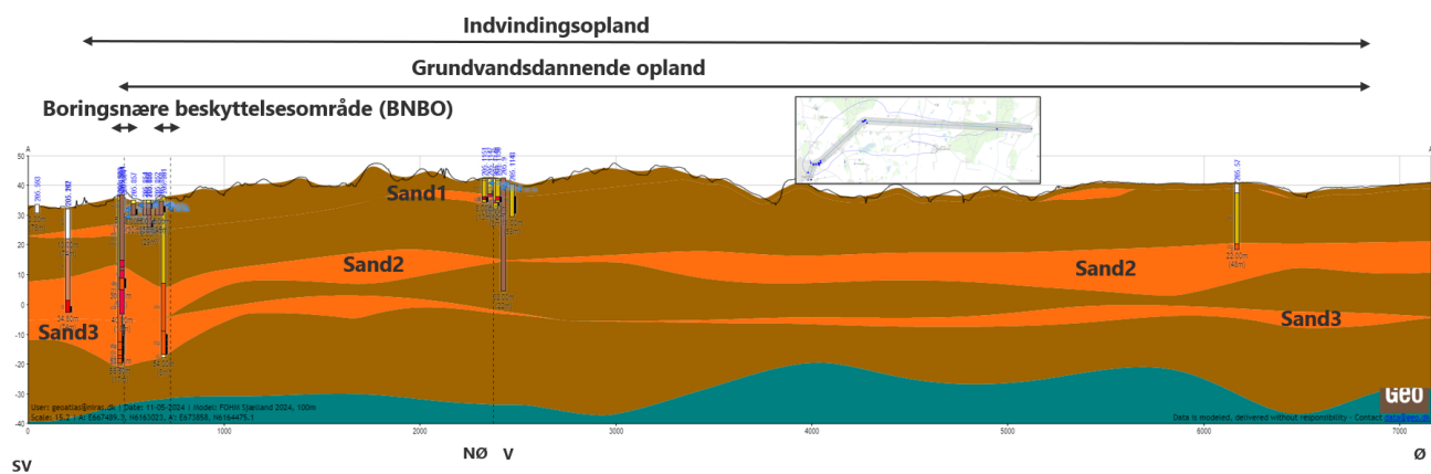
Figur 64 Geologisk profil gennem kildepladserne. Brune og blå farver repræsenterer vandstandsene og oftest lerede aflejringer, orange og grønne farver repræsenterer vandførende aflejringer, typisk sand og grus eller kalk.
