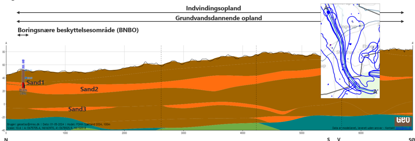
Figur 3 Geologisk profil gennem kildepladsen. Brune og blå farver repræsenterer vandstandsede og oftest lerede aflejringer, orange og grønne farver repræsenterer vandførende aflejringer, typisk sand og grus eller kalk.
