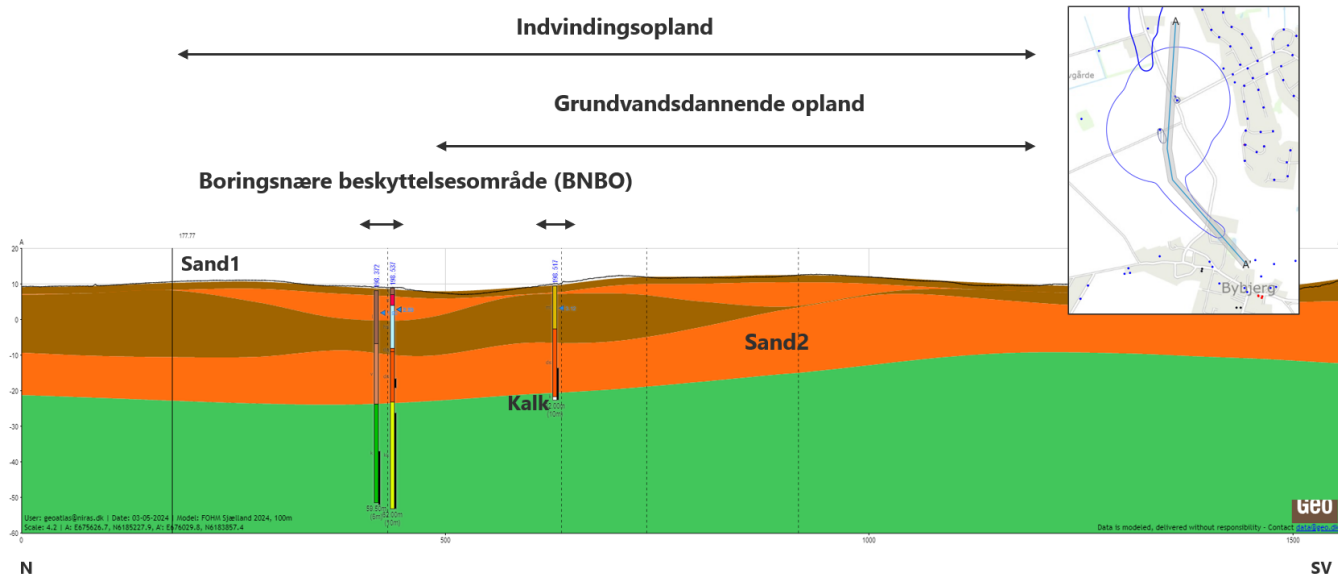
Figur 36 Geologisk profil gennem kildepladsen. Brune farver repræsenterer vandstandsende og oftest lerede aflejringer, orange farver repræsenterer vandførende aflejringer, typisk sand og grus. Den grønne farve viser kalken.
