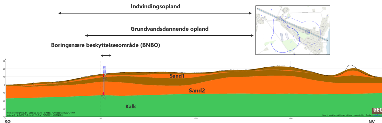
Figur 20 Geologisk profil gennem kildepladsen. Brune farver repræsenterer vandstandsende og oftest lerede aflejringer, orange farver repræsenterer vandførende aflejringer, typisk sand og grus. Den grønne farve viser kalken.
