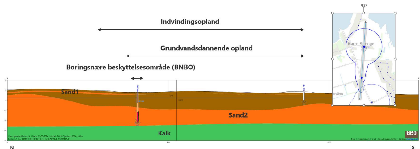
Figur 12 Geologisk profil gennem kildepladsen. Brune farver repræsenterer vandstandsende og oftest lerede aflejringer, orange farver repræsenterer vandførende aflejringer, typisk sand og grus. Den grønne farve viser kalken.
