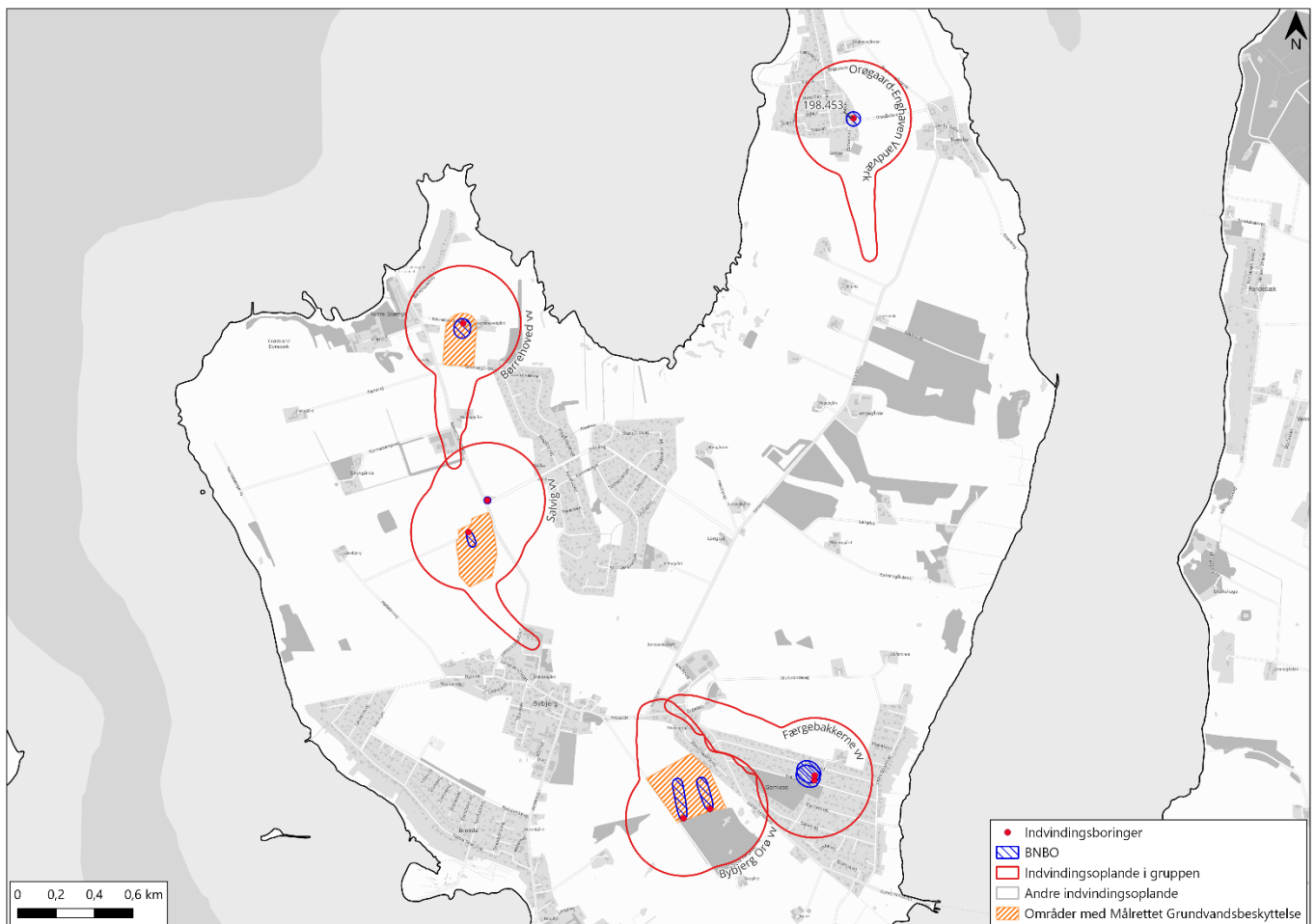
Figur 1 Kortet viser de 5 kildepladsers aktive indvindingsboringer, BNBO, indvindingsopland og områder med målrettet grundvandsbeskyttelse.
