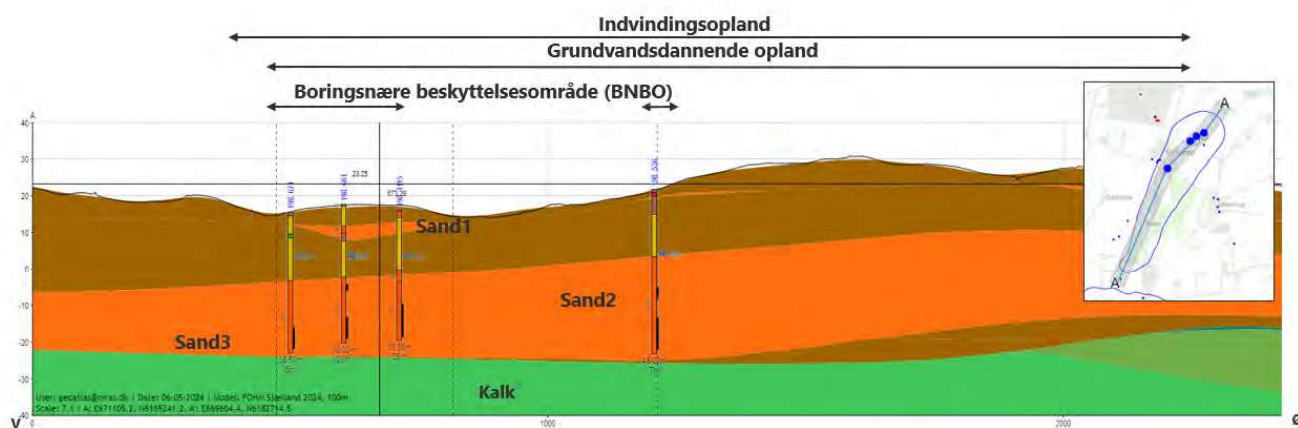
Figur 11 Geologisk profil gennem kildepladserne. Brune farver repræsenterer vandstandsende og oftest lerede aflejringer, orange farver repræsenterer vandførende aflejringer, typisk sand og grus.
