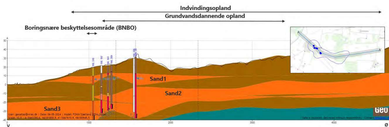
Figur 3 Geologisk profil gennem kildepladsen. Brune farver repræsenterer vandstandsede og oftest lerede aflejringer, orange farver repræsenterer vandførende aflejringer, typisk sand og grus. Den grønne farve viser kalken.
