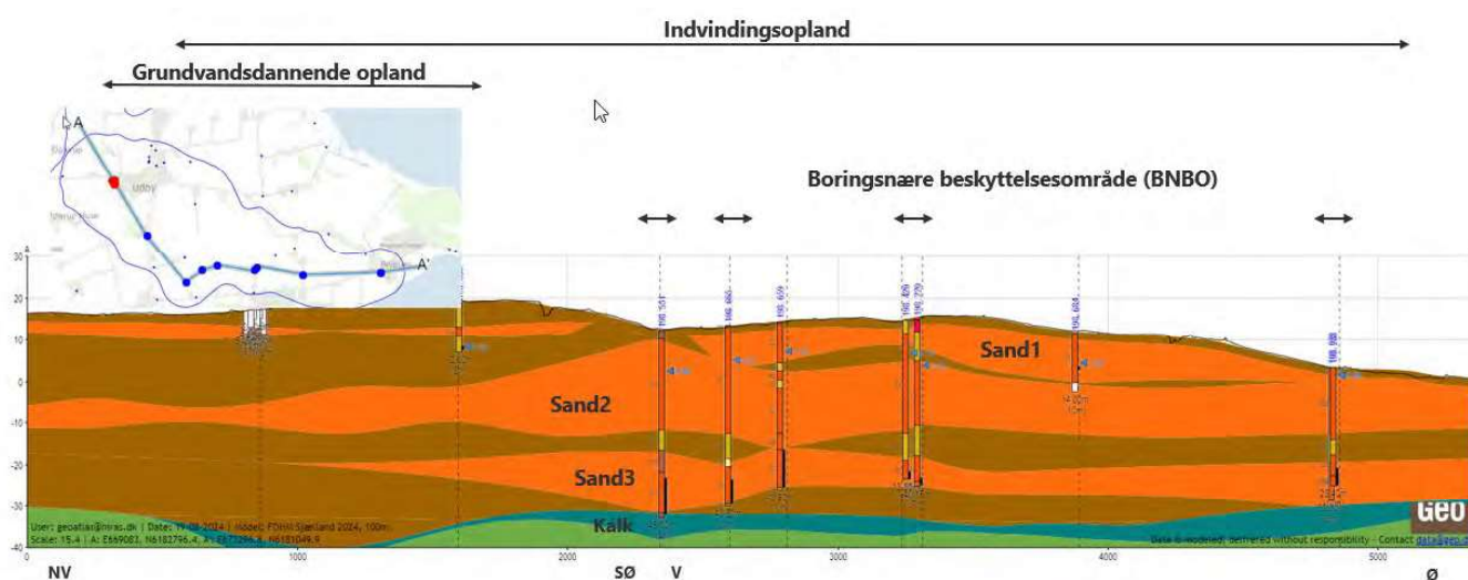
Figur 27 Geologisk profil gennem kildepladserne. Brune farver repræsenterer vandstandsede og oftest lerede aflejringer, orange farver repræsenterer vandførende aflejringer, typisk sand og grus.
