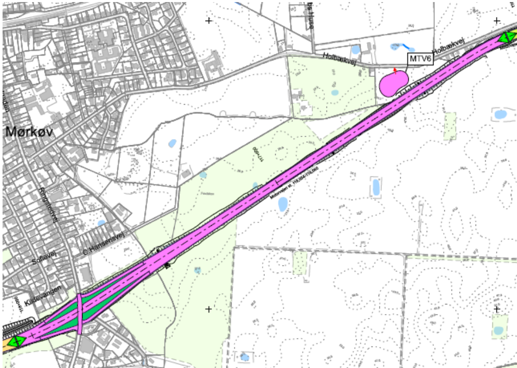
Figur 2. Kortudsnit over strækningen af Kalundborgmotorvejen som ledes til MTV6 (markeret med lyselilla). Fra MTV6 ledes det rensede og forsinkede vand til tilløb til Egemoseløbet via udledningspunktet 585644.30, 1169837.57 beliggende nord for motorvejen.
