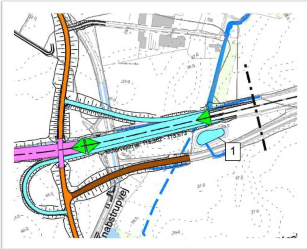
Figur 2. Kortudsniit over strækningen af Kalundborgmotorvejen som ledes til Bassin 1 (markeret med lyseblåt). Fra Bassin 1 ledes det rensede og forsinkede vand til Tuse Å via udledningspunktet 588613.91, 1170424.2 beliggende mellem motorvejen og tilkørselsrampe.
